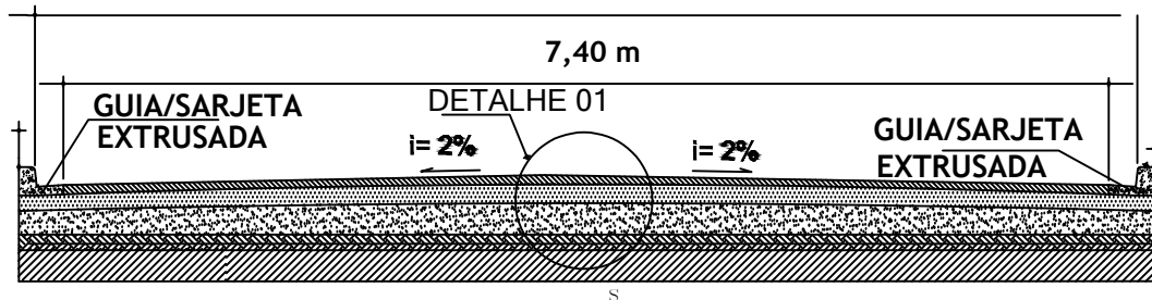
CORTE TRANSVERSAL - PISTA DE ROLAMENTO INTERTRAVADO E = 8,0 CM
